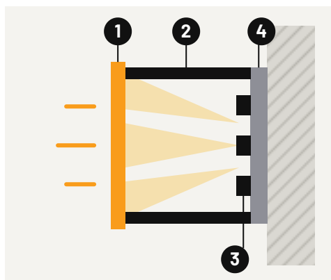
Corte lateral de una letra
