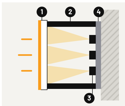
Corte lateral de la caja
