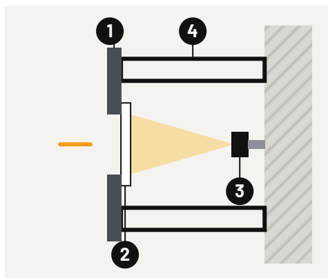
Corte lateral, versión calada con luz
